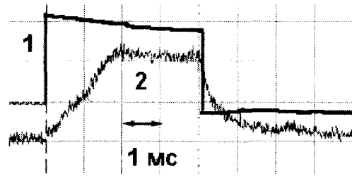
Рис. 2. Совмещенная осциллограмма напряжения и тока типовой форсунки: 1 - напряжение; 2 - ток
