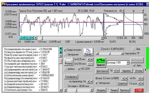
Рис. 2. Профилограмма поверхности ролика и параметры шероховатости ее поверхности
