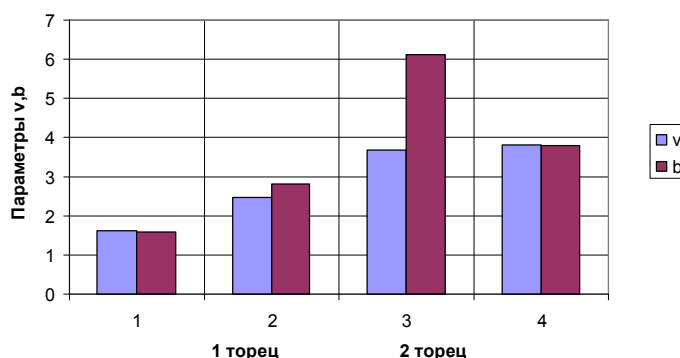
Рис. 8. Параметры относительной опорной поверхности торцов роликов
