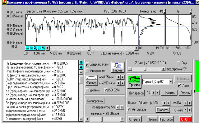
Рис. 5. Шероховатость поверхности торца ролика 1 в радиальном направлении
