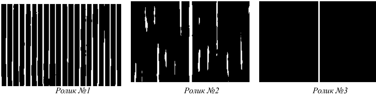
Рис. 16. Бинарные изображения двумерных автокорреляционных поверхностей для r=0,61
