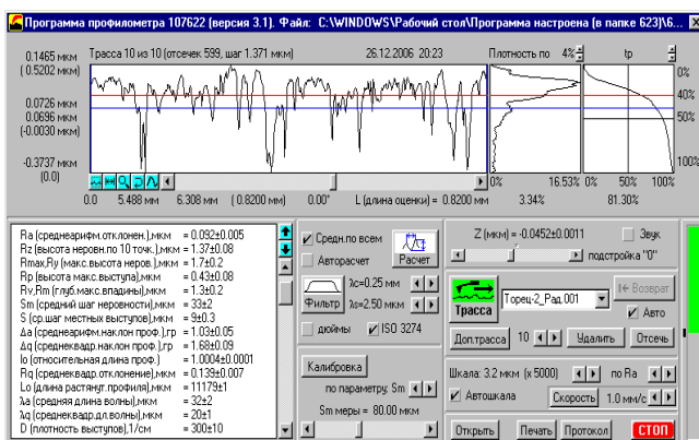
Рис. 6. Шероховатость поверхности торца ролика 2 в осевом направлении
