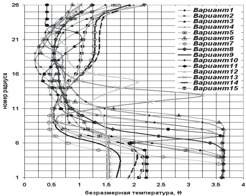
Рис. 6. Радиальная эюра безразмерной температуры, осредненной в окружном направлении на расстоянии 2d от последнего ряда отверстий, d – диаметр отверстия в первом ряду
