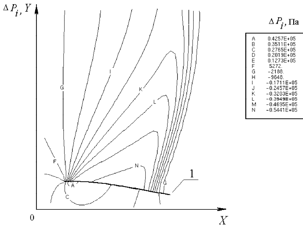
Рис. 7. Изобары у профиля крыла 1
