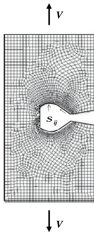
Рис. 2. Упругопластическая часть полосы
