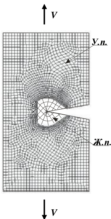
Рис. 1. Схема применения суперэлемента в задаче о растяжении полосы
