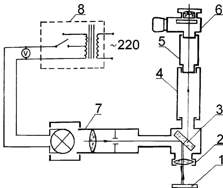
Рис. 1. Схема устройства освещения компаратора ИЗА-2
