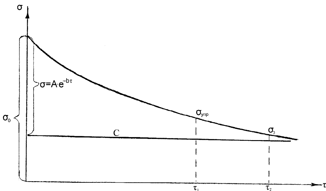
Рис. 2. График изменения остаточных напряжений
