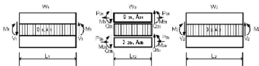
Рис. 2. Модель сотовой конструкции с отслоением обшивки а) модель трёхслойной конструкции; б) модель трёхслойной конструкции с отслоением
