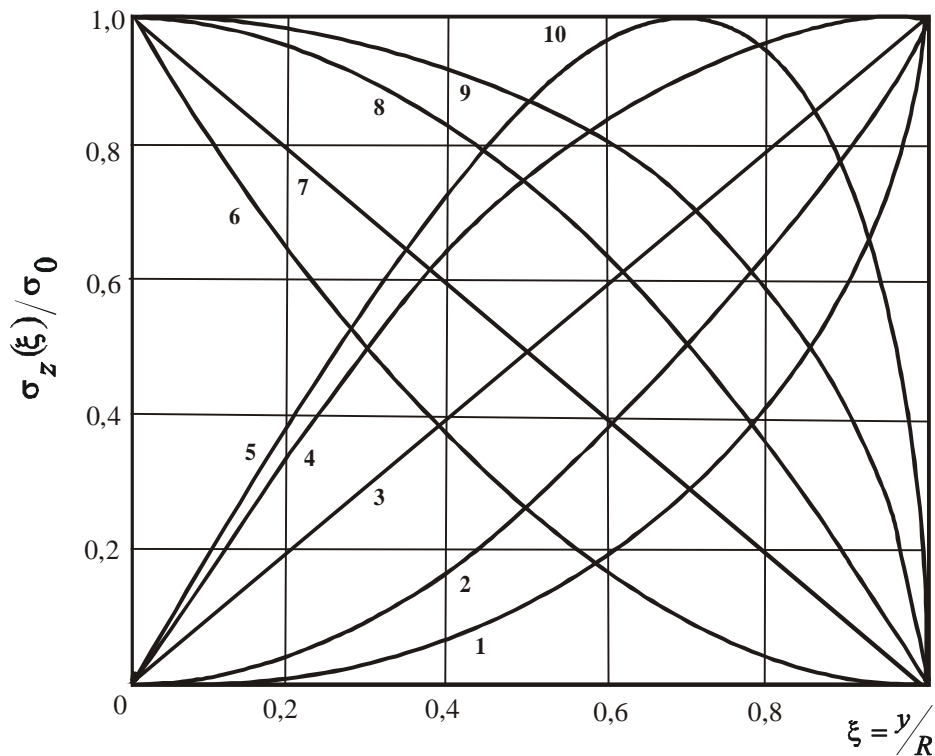
Рис. 2. Варианты распределения остаточных напряжений гладкой детали
