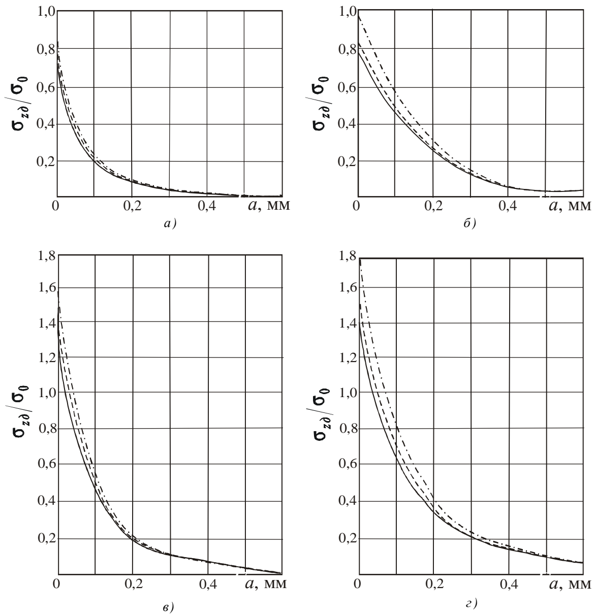
Рис. 4. Дополнительные осевые остаточные напряжения в наименьшем сечении сплошных (—) и полых (--- d=10 мм, - x - d=12 мм) деталей диаметром D=15 мм с надрезом R=0,3 мм для вариантов табл. 1: а – 1, б – 7, в – 3, г – 9
