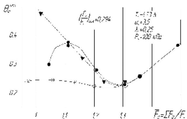
Рис. 5. Влияние раскрытия жаровой трубы на \theta_j^{\text{max}} камеры сгорания двигателя МД-120:
