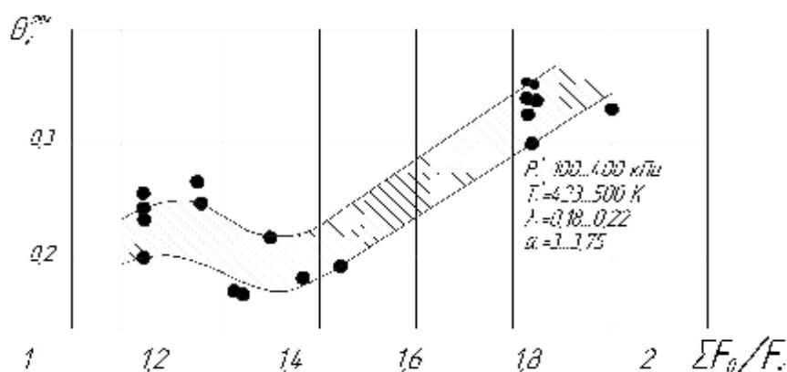
Рис. 6. Влияние отношения \Sigma F_0 / F_k на характеристики выходного поля температур газа КС двигателя МД-45
