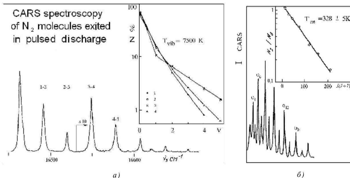
Рис. 2. Спектры колебательно-вращательных переходов молекул азота, возбужденных в разряде, и соответствующие функции распределения по колебательным (а) и вращательным (б) уровням энергии
