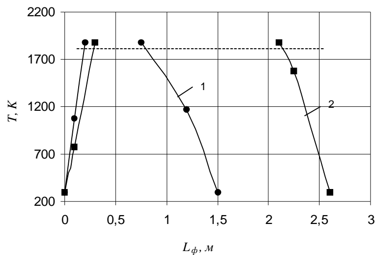
Рис. 6. Зависимость температуры на оси факела от параметра закрутки S и формы насадки: горючее - АСД-4 + АПС-1 + ПА-1 (в соотношении 10:5:4 по объему); a = 2,4 ; M = 0,4 ; 1 - диффузная насадка ( S = 2,0 ); 2 - цилиндрическая насадка ( S = 1,8 )
