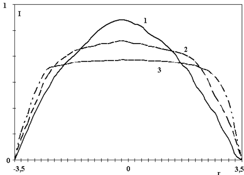
1 – неискривленная поверхность, 2 – поверхность с отрицательным радиусом кривизны, 3 – поверхность с положительным радиусом кривизны
