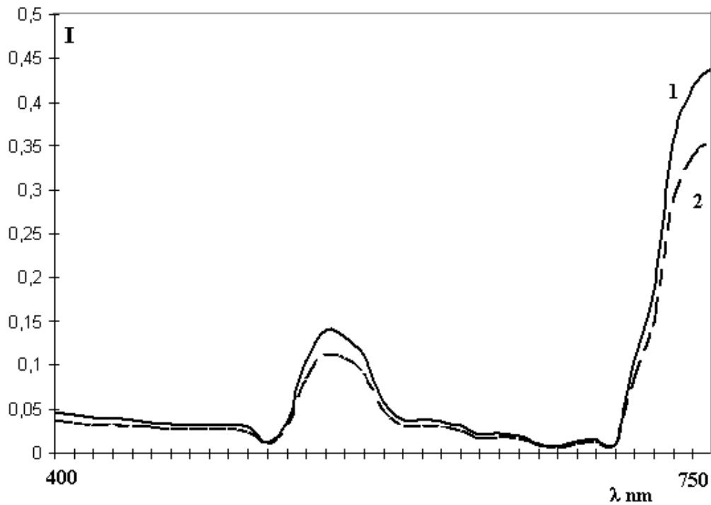
1 – гладкая поверхность без неоднородностей; 2 – модель «синуса» Рис. 3. Спектры нормированной интенсивности обратного рассеяния I(\lambda) для различных моделей поверхности
