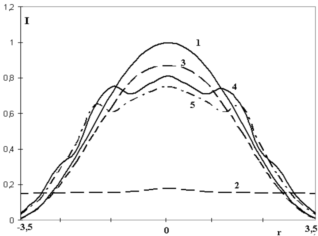
1 - зеркальная поверхность, 2 – матовая поверхность, 3 – гладкая поверхность без неоднородностей, 4 – модель «синуса», 5 – модель «цилиндров» Рис. 4. Радиальное распределение нормированной интенсивности I(r) обратного рассеяния
